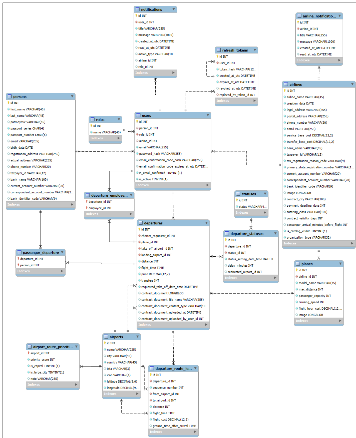
Рисунок В.1 – ER диаграмма БД
