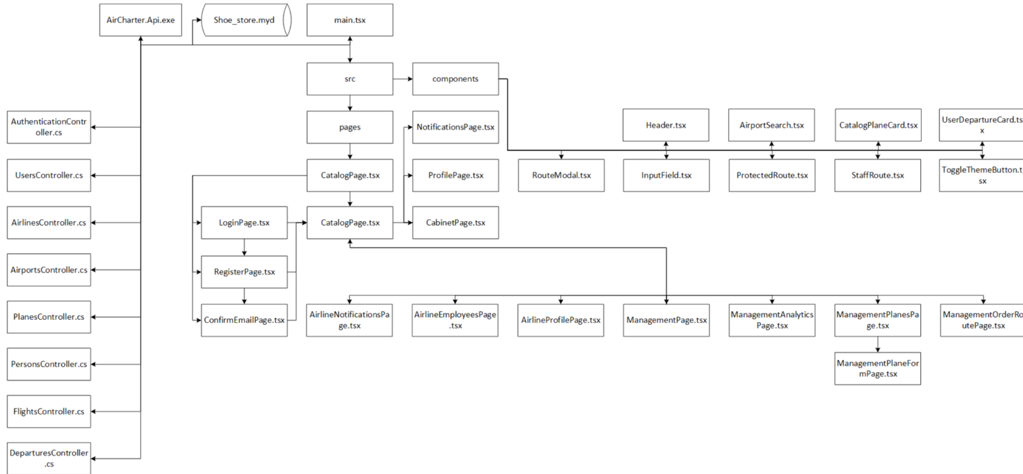
Рисунок Г.1 – Модульная схема приложения
