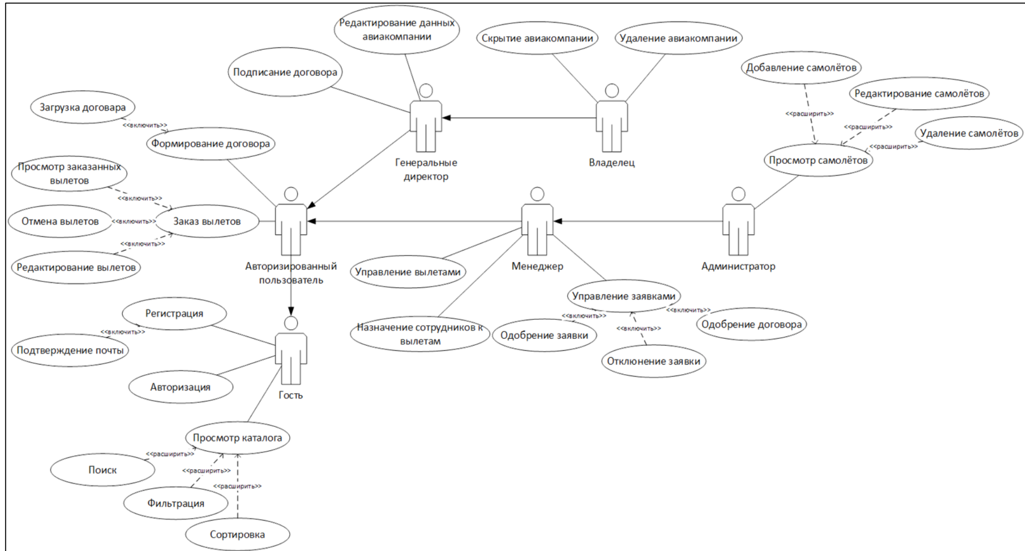
Рисунок А.1 – Диаграмма вариантов использования
